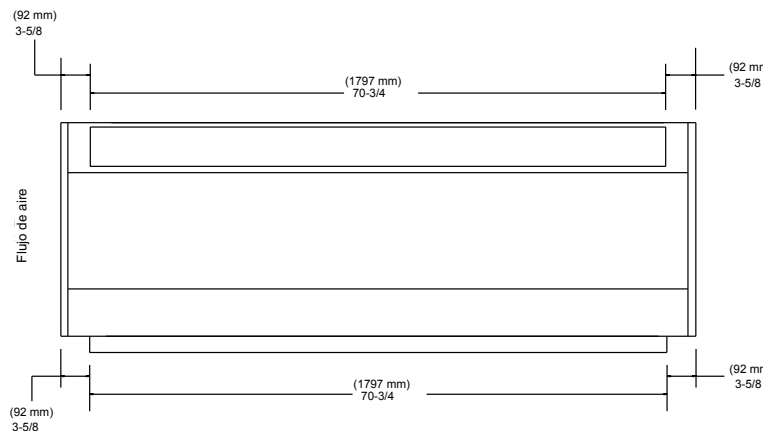
VISTA FRONTAL GABINETE DE 1981 mm (78 PULG.)
