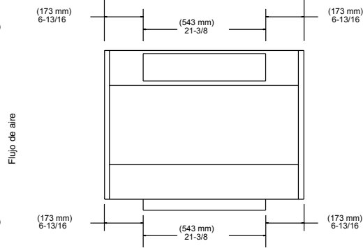
VISTA FRONTAL GABINETE DE 889 mm (35 PULG.)
