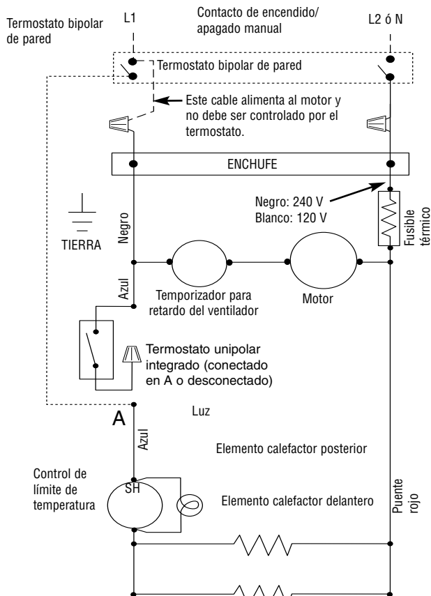
Figura 3 – Conexión del termostato remoto (si desea la menor potencia, desmonte el puente rojo)
